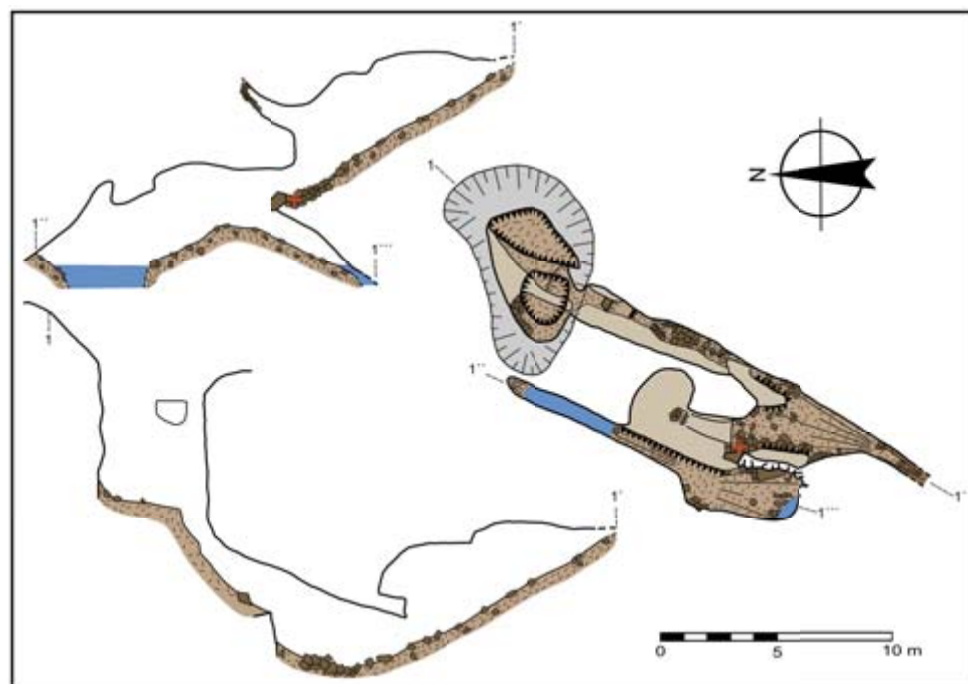
Obr. 1 | Mapa Dvojité šachty, křížkem vyznačena poloha datované vrstvy uhlíků. Podle Cíchy (1992, 1993).
