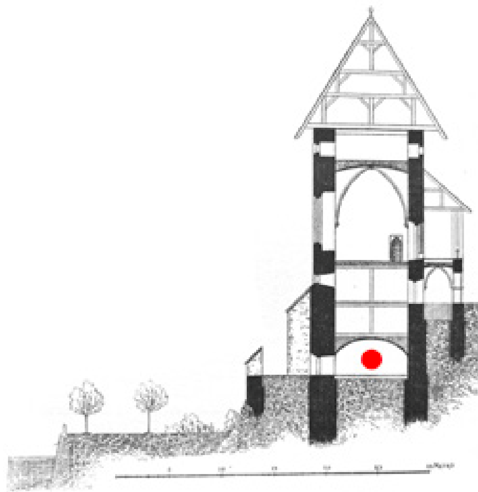
Obr. 1 | Řez západním křídlem hradu s vyznačením suterénu (podle A. Sedláčka 1913)
