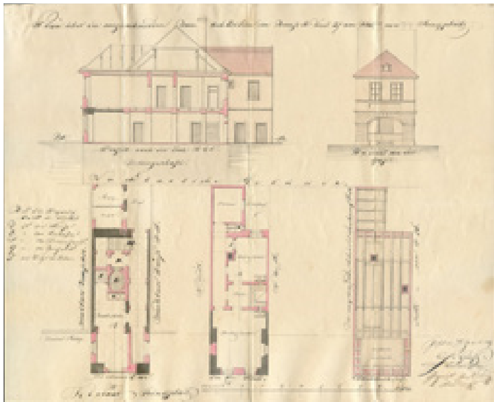
Obr. 9 | Plán přestavby domu čp. 37 na Malém rynku od píseckého stavitele Františka Spiesse ze 7. dubna 1839. Státní okresní archiv Písek, Archiv města Písek, kart. 1546, sig. D IV 22 č. d. 37.
