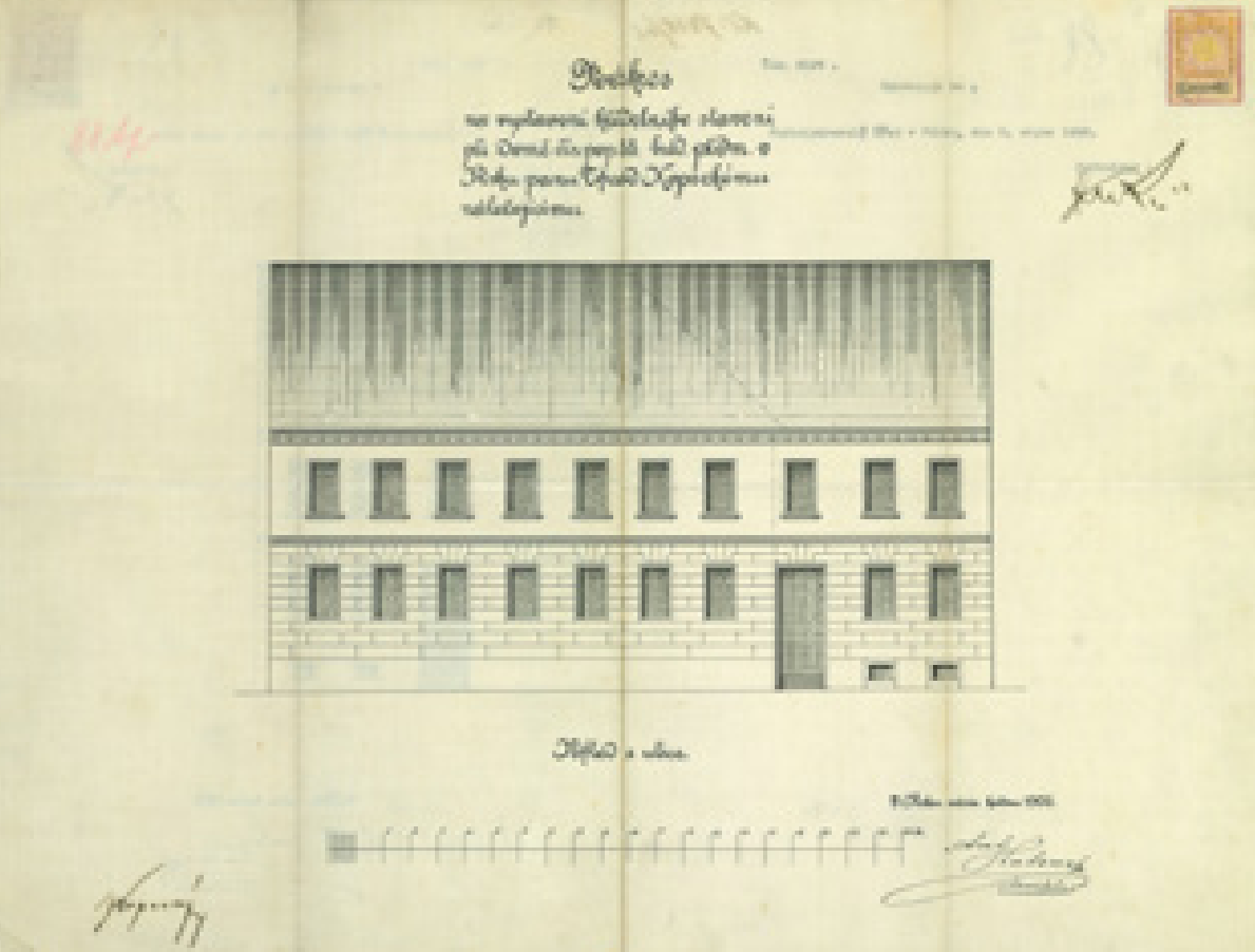
Obr. 4 | Návrh nové fasády po dostavbě čp. 88 o Kopeckého tiskárnu a ubourání vstupního schodiště. Městský úřad Písek, archiv odboru výstavby a územního plánování, složka domu čp. 88 – Budějovické předměstí.
